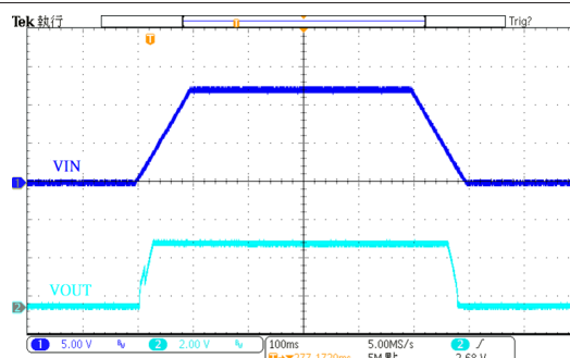
电源 ON/OFF 响应 HT75H33
