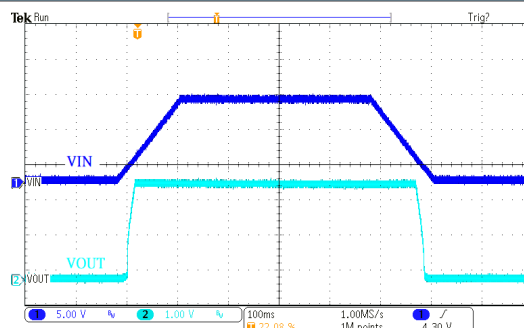
电源 ON/OFF 响应 HT75H27
