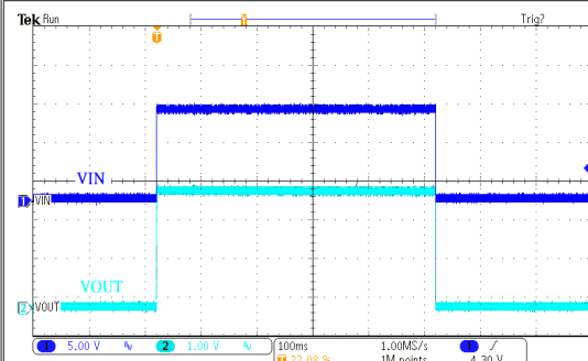
电源 ON/OFF 响应 HT75H30
