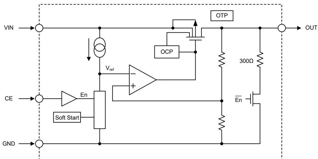
方框图
