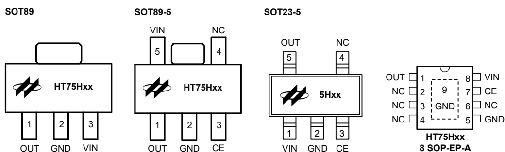
引脚图
