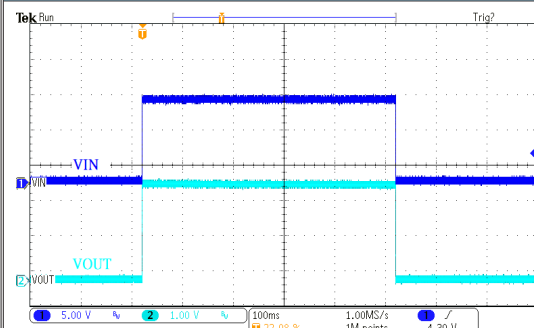
电源 ON/OFF 响应 HT75H27
