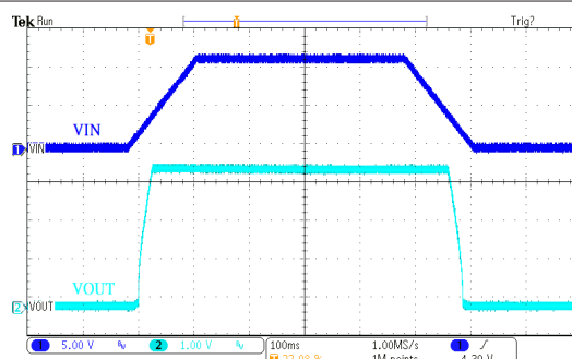
电源 ON/OFF 响应 HT75H36
