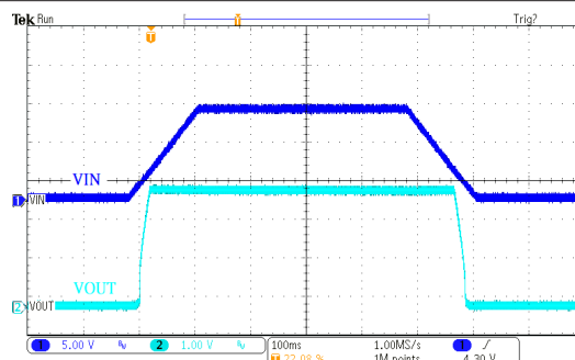
电源 ON/OFF 响应 HT75H30
