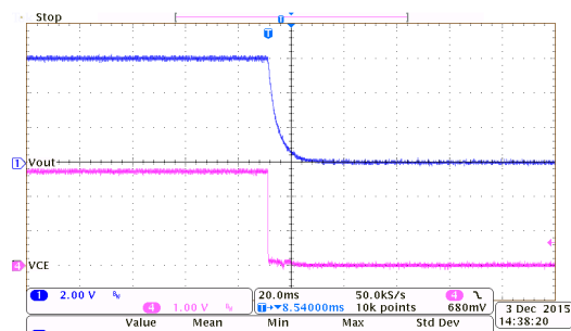
开关响应: HT7560-7 ( I_{OUT}=150mA , V_{CE}=2.7V to 0V)
