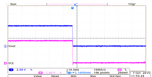
开关响应: HT7550-7 ( I_{OUT}=150mA , V_{CE}=2.7V to 0V)
