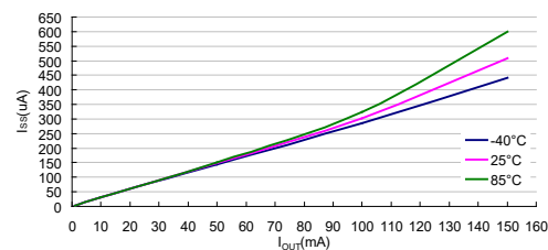
I_{SS} vs I_{OUT} : HT75C0-7 ( V_{IN}=14V )
