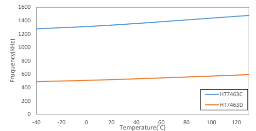
f SW vs. TEMP (HT7463C 和 HT7463D)
